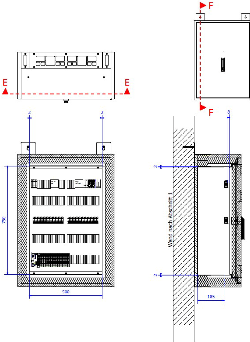
Schnitt E-E
